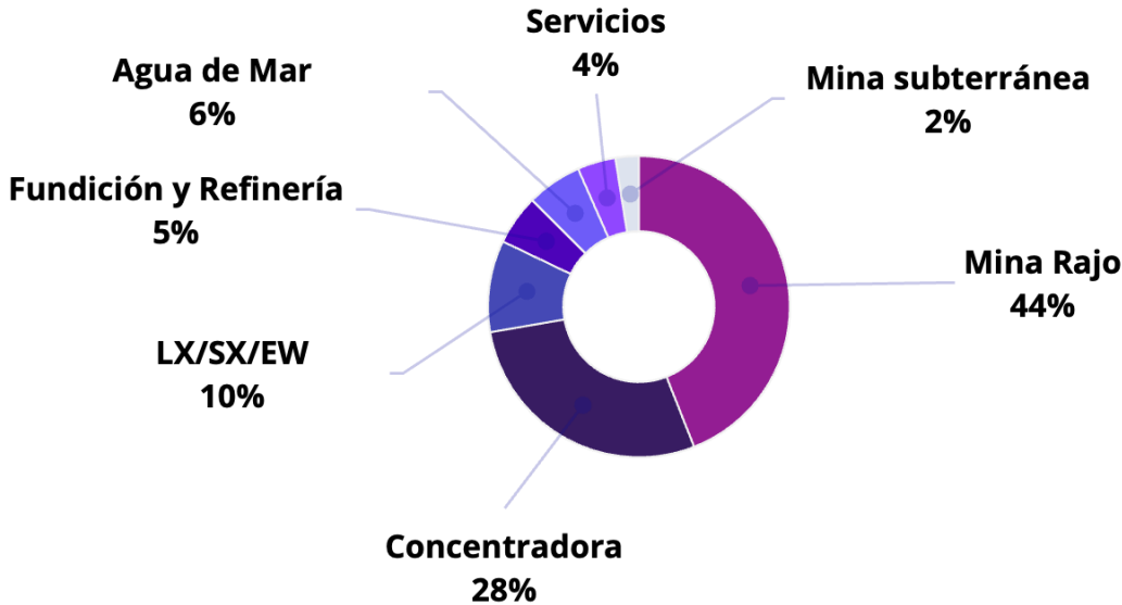
Consumo energético por procesos Total 210.619 TJ
