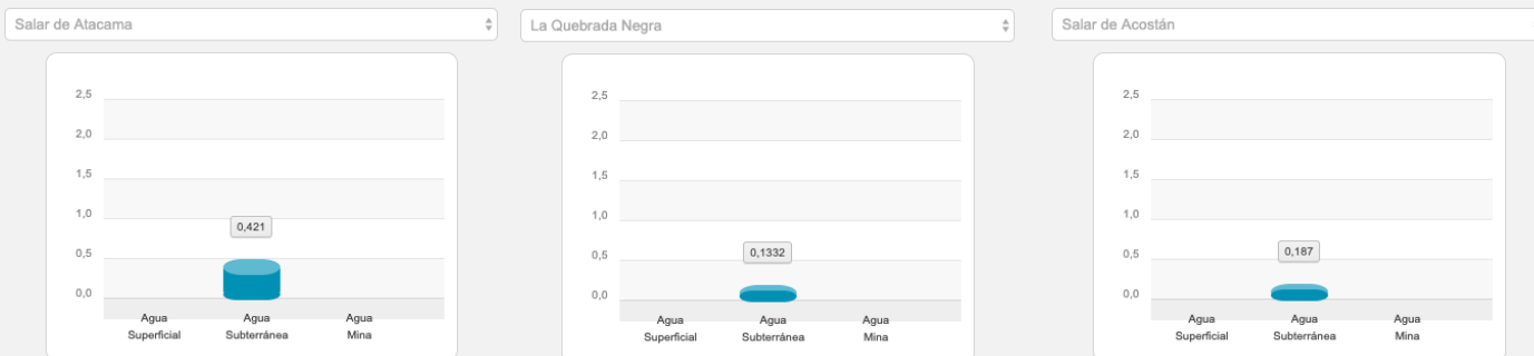
Extracción de agua Región de Antofagasta Gran Minería 2018, por cuenca (m3/s)
