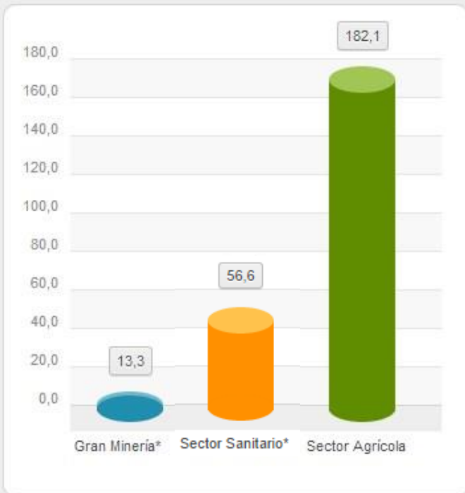
Extracción de agua regiones I a VI por sector año 2012 (m3/s)
