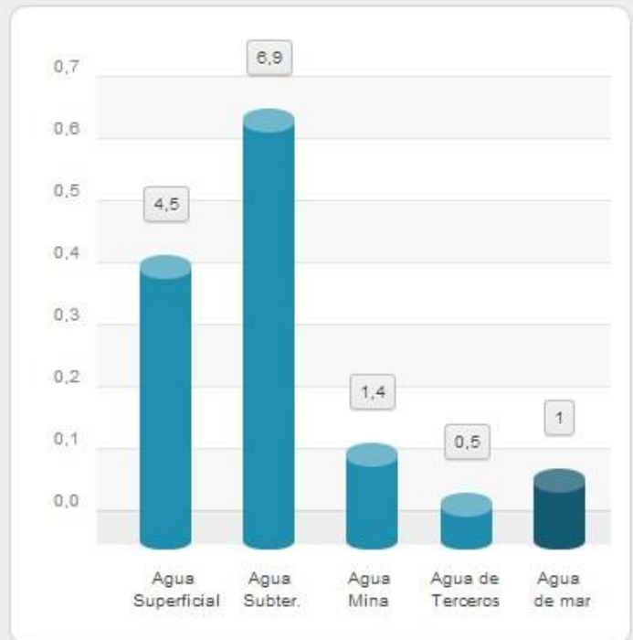
Extracción de agua regiones I a VI Gran Minería año 2012 (m3/s)
